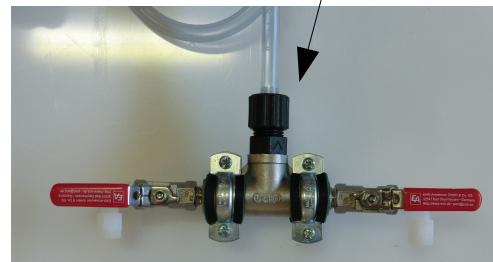
2x 2-Wege-Hahn zum auswählen eines Dosierbehälters
